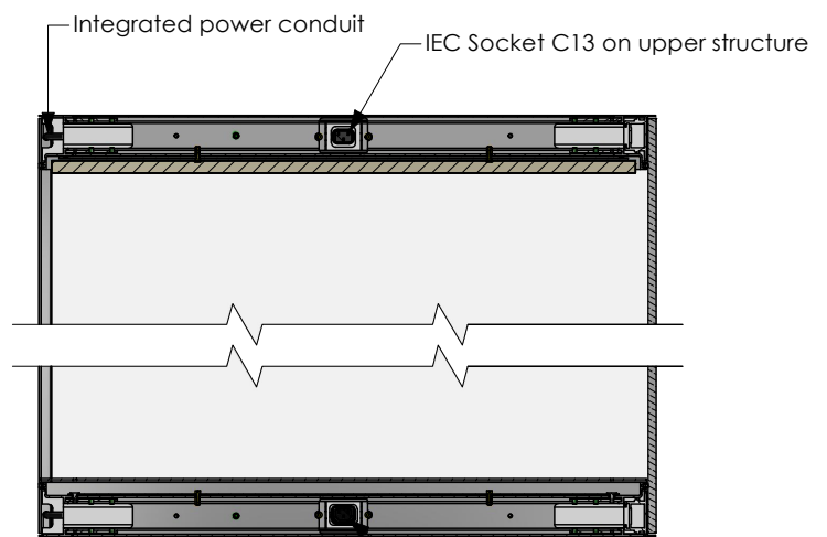
G POWER CONDUIT DETAIL
