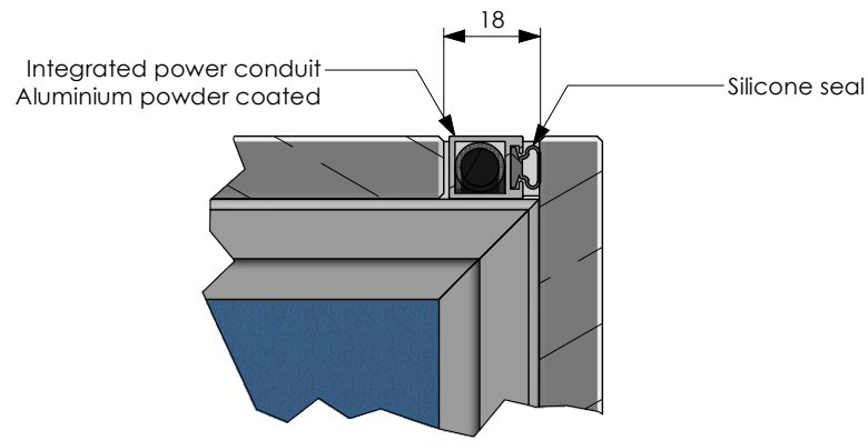
G POWER CONDUIT DETAIL
